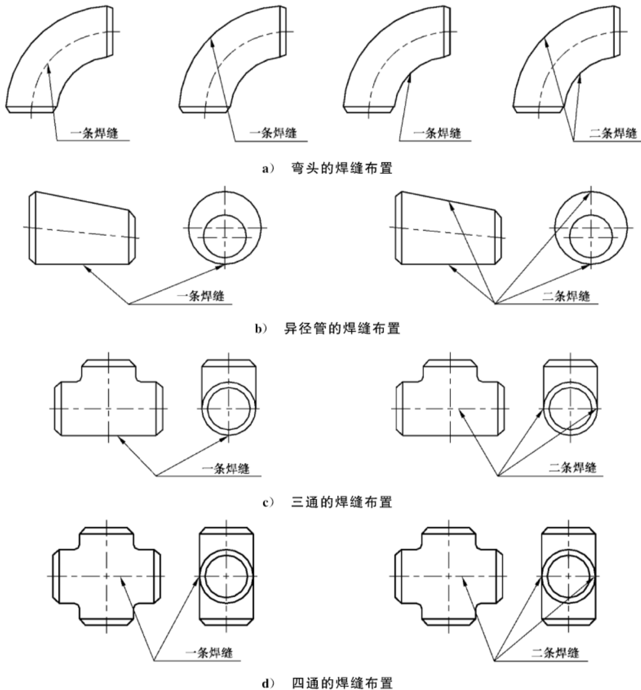
图 1 焊接管件的焊缝布置示意图
